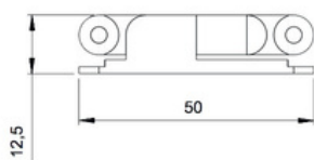
Afmetingen handgreep
