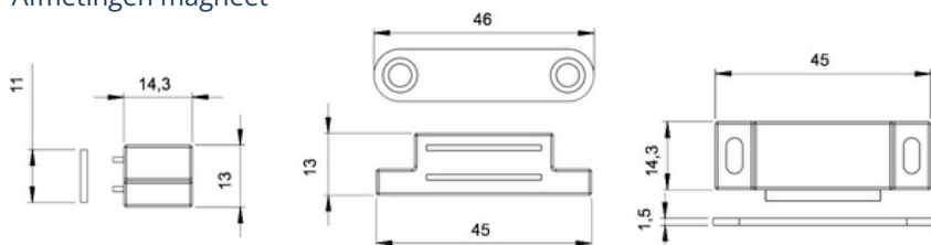
Afmetingen magneet
